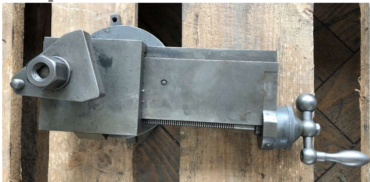
Chariot IMG_2914 - CHF 220.—
